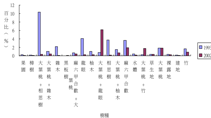
圖 48 新化林場 1993-2002 年最大嵌塊比變化
