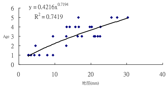
圖 35 疏伐度 10%之地徑與林齡關係
