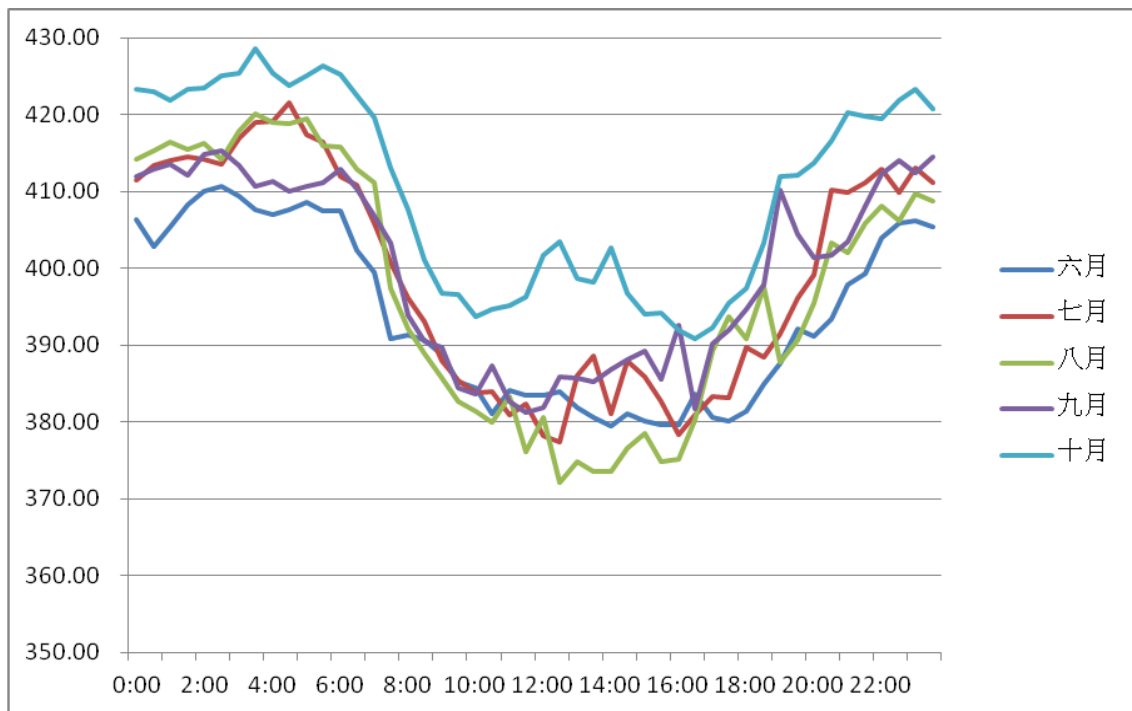
圖 4 屏東觀測站 2011 年各月份大氣二氧化碳濃度日變化。
