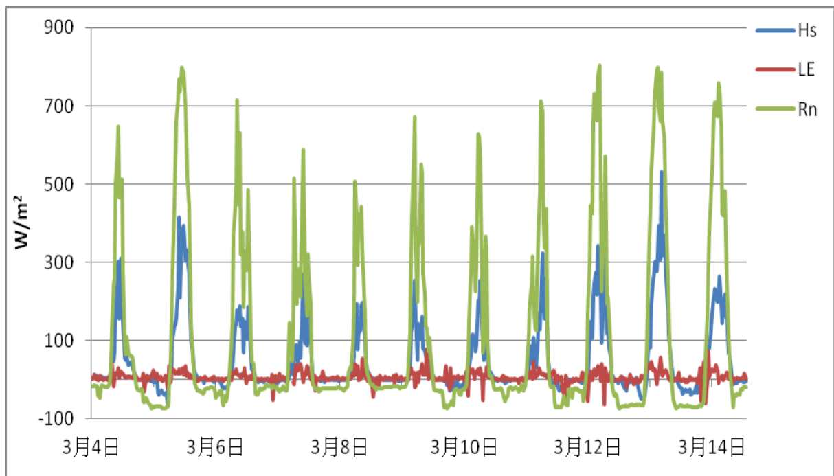
圖 5 屏東地區各項通量整合圖(以 2011 年 3 月 4~14 日為例)
