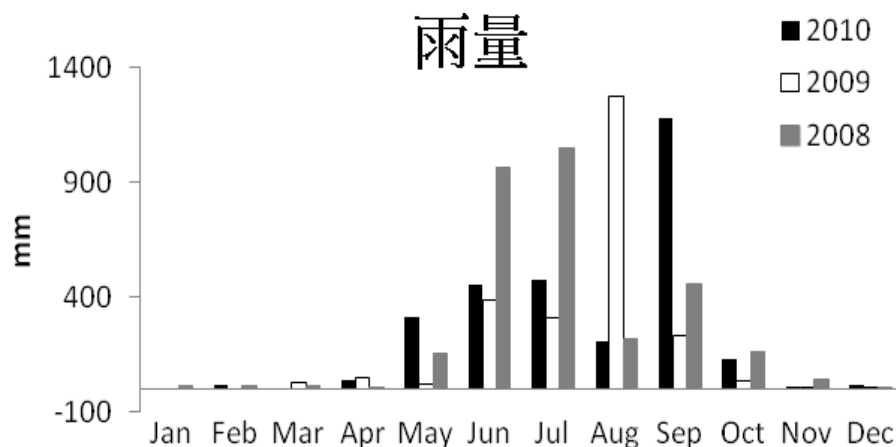
圖 6 屏東地區 2008-2010 年月雨量變化
