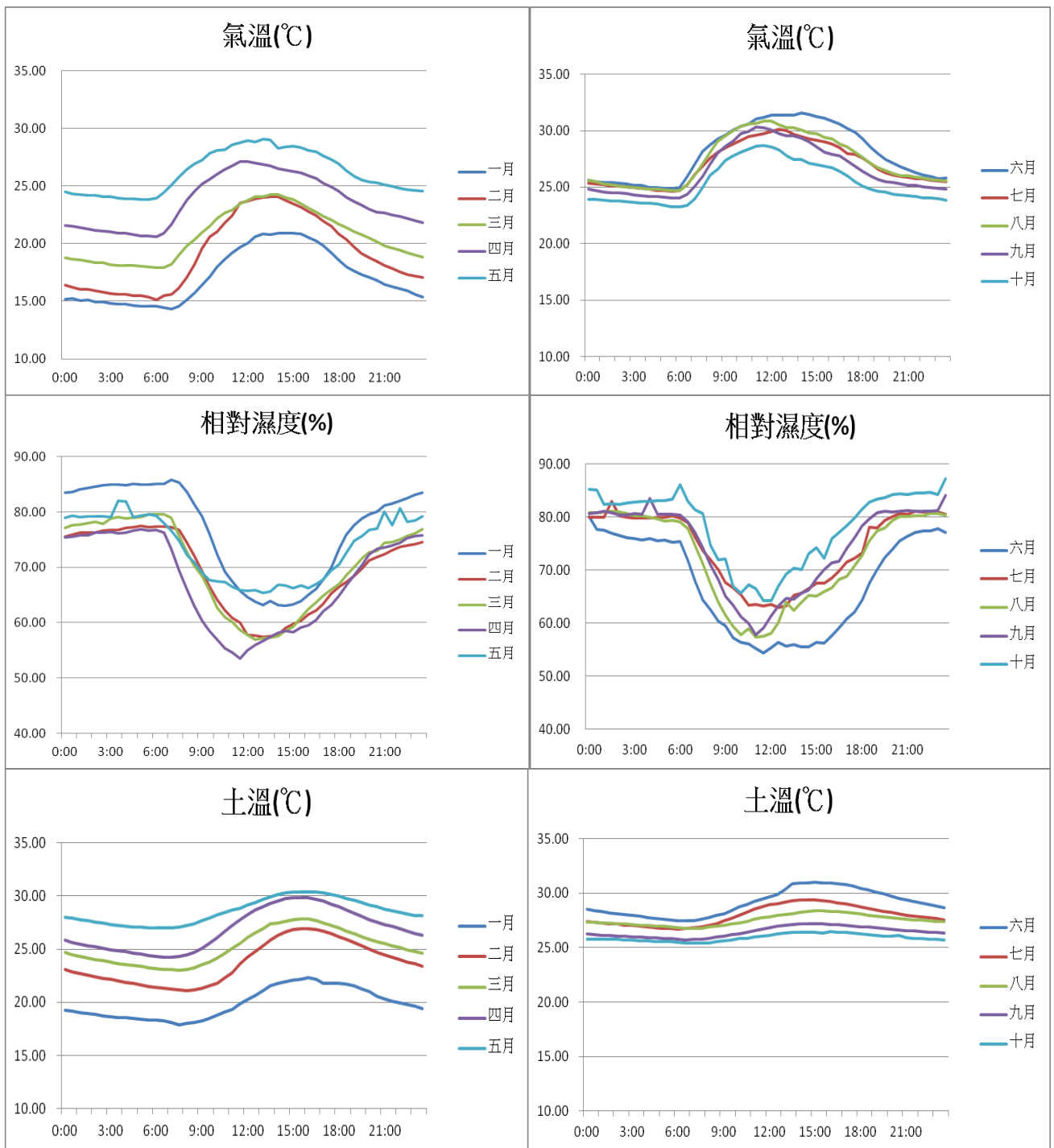
圖 7 2011 年一月至十月屏東觀測站微氣候資料。
