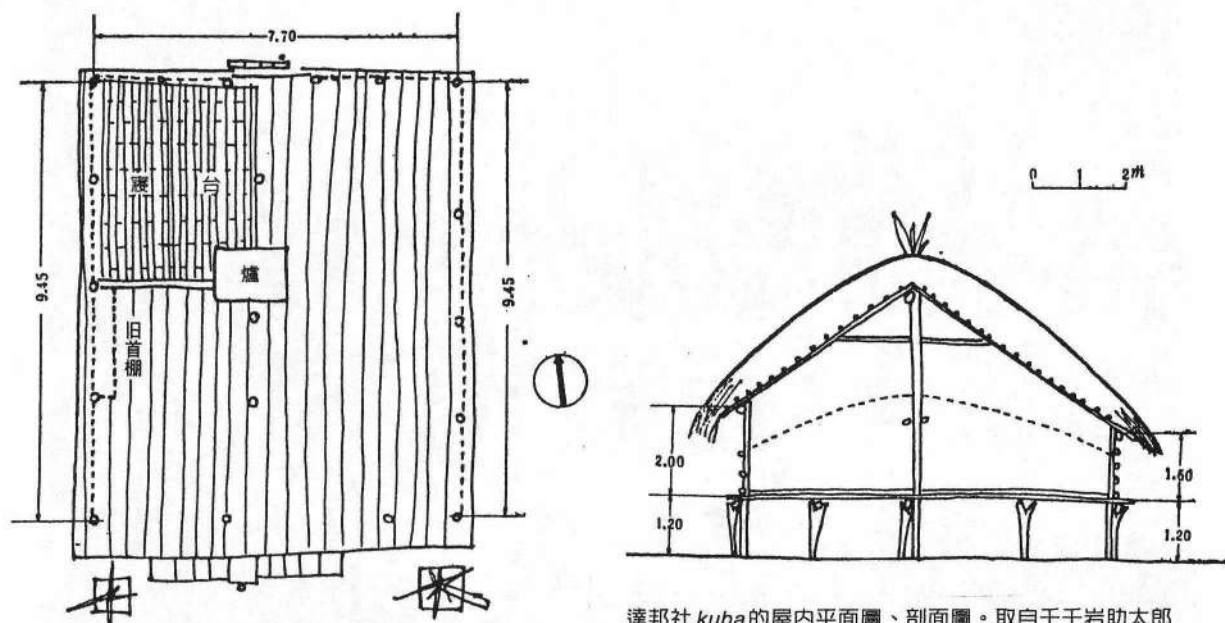
達邦社 kuba 的屋內平面圖、剖面圖。取自千千岩助太郎「台灣高砂族の住家」(1960)。
