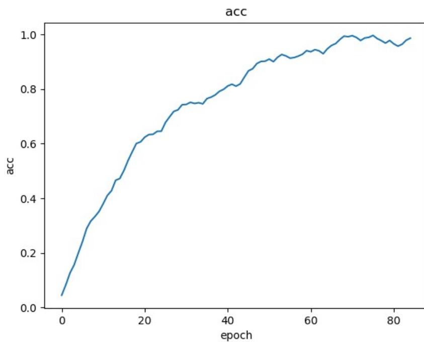
圖 5-4 模型訓練精度(acc)與迭代訓練週期(epoch)關係圖
