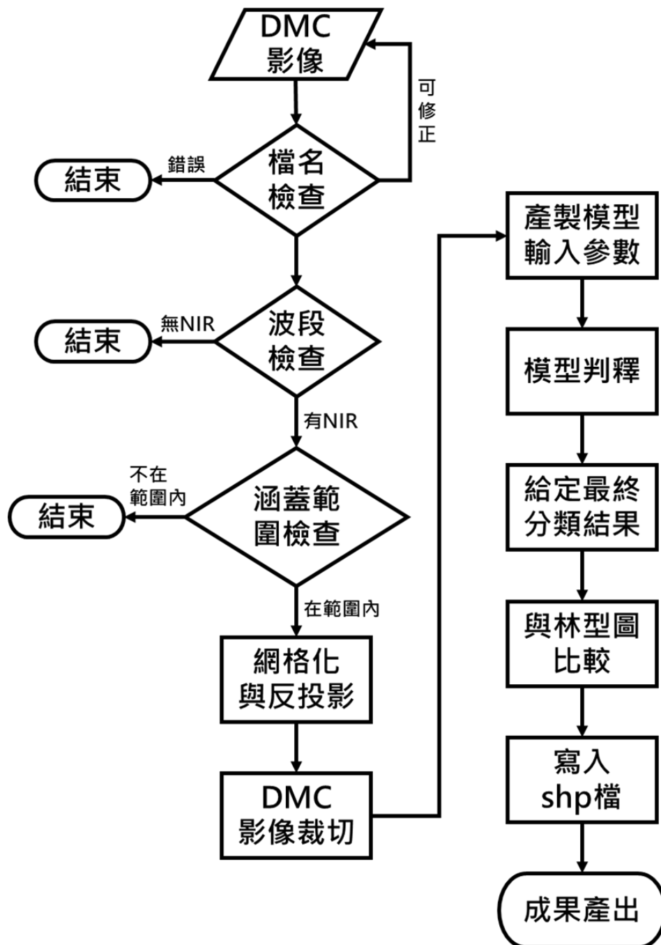
圖 4-14 森林覆蓋型辨識工具運作流程
