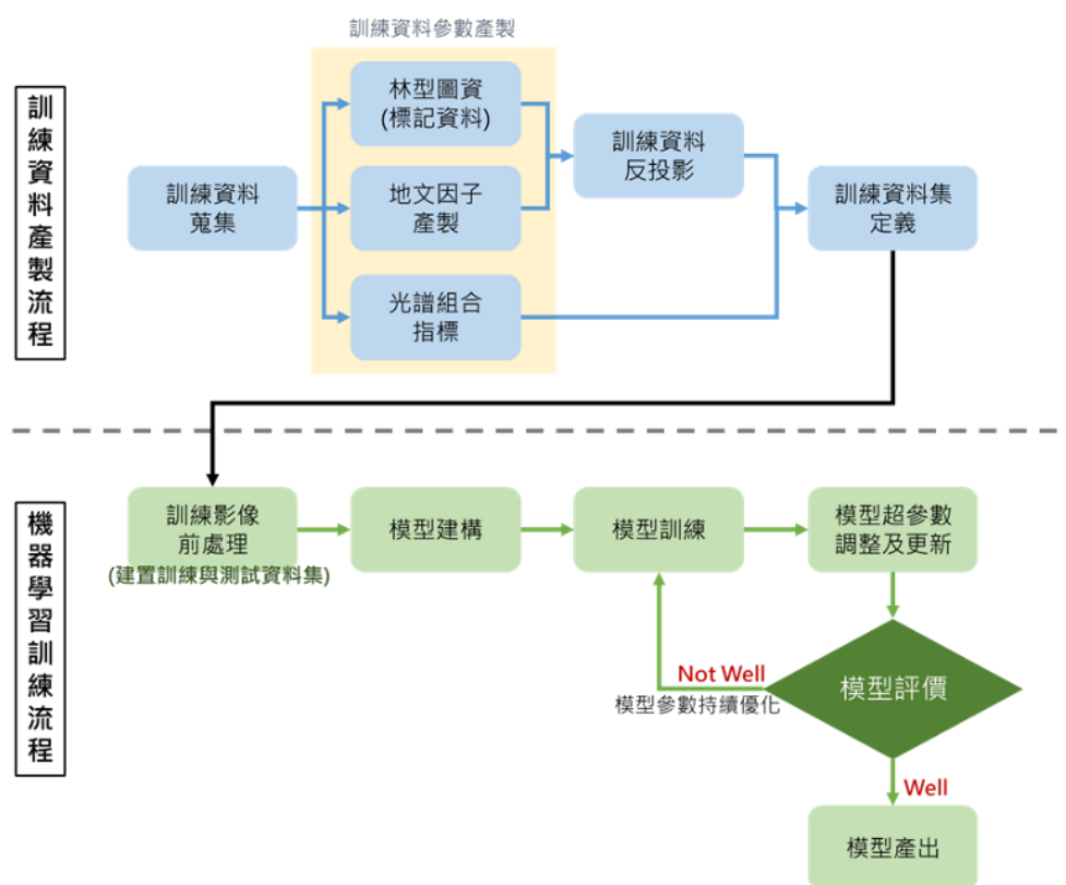
圖 6-1 機器學習訓練流程
