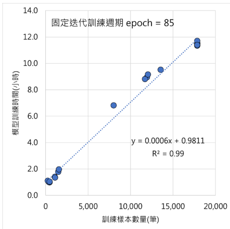
圖 5-2 模型訓練時間與樣本數量關係圖
