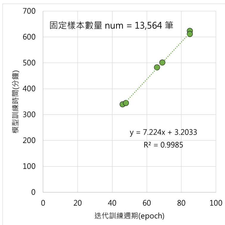
圖 5-3 模型訓練時間與迭代訓練週期關係圖
