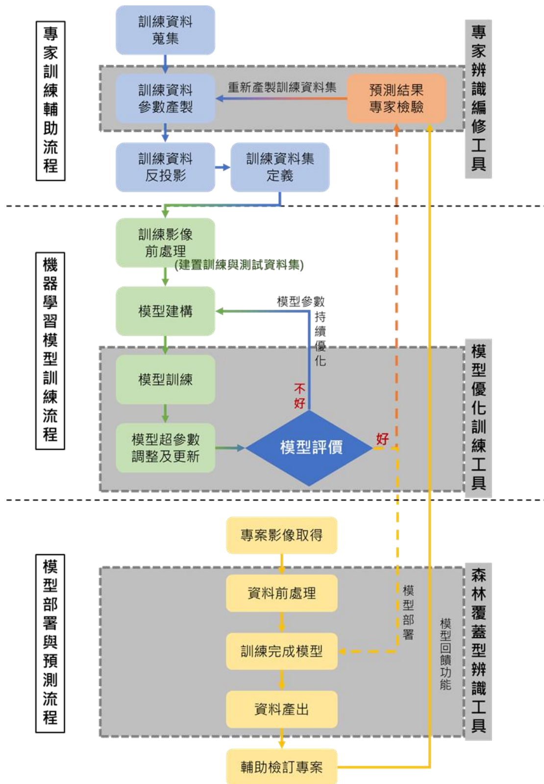
圖 4-1 機器學習架構流程與工具扮演角色
