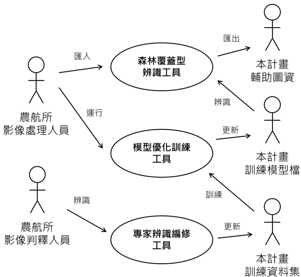
圖 4-5 本計畫 111 年度規劃機器學習工具案例圖
