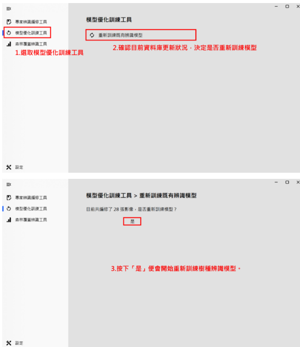
圖 4-12 模型優化訓練工具畫面
