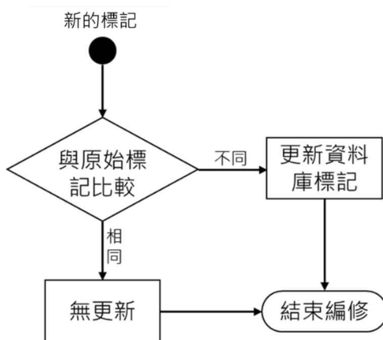
圖 4-8 專家辨識編修工具運作流程
