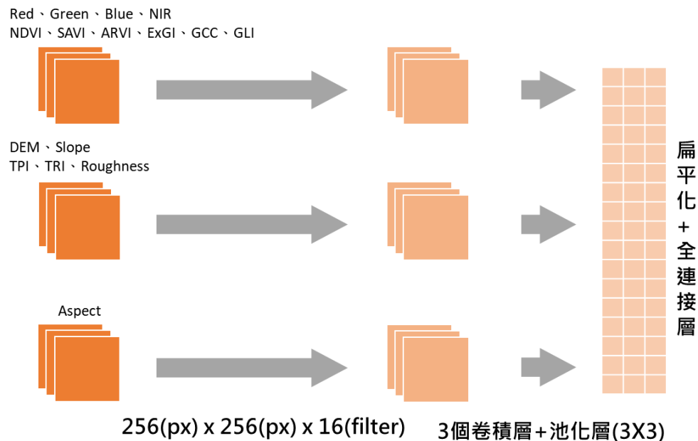
圖 6-2 特殊樹種銀合歡辨識模型架構
