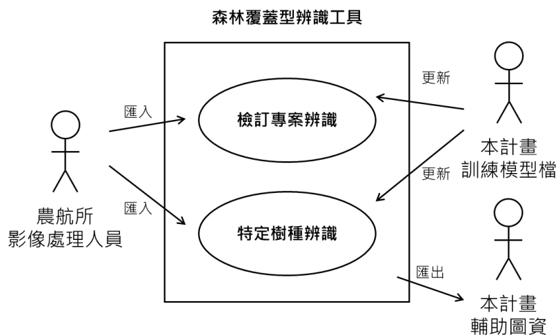
圖 4-4 森林覆蓋型辨識工具案例圖
