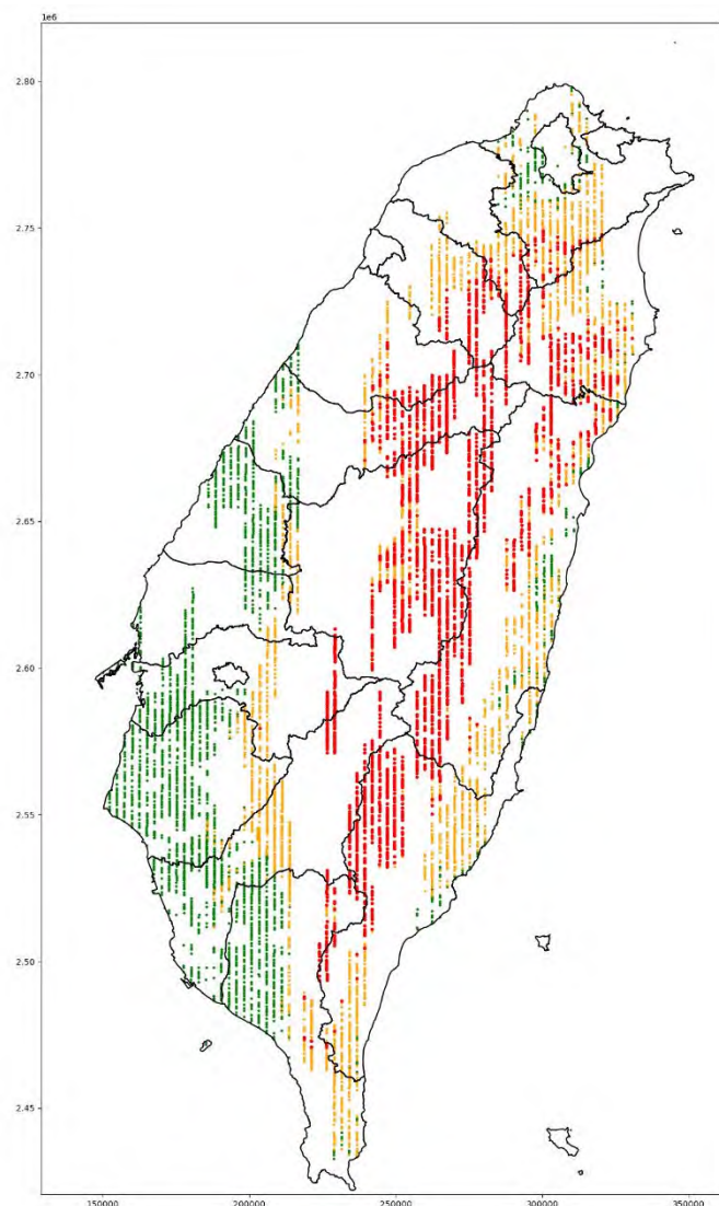
圖 3.8 驗證資料集的 8000 張航攝原始影像分布圖
