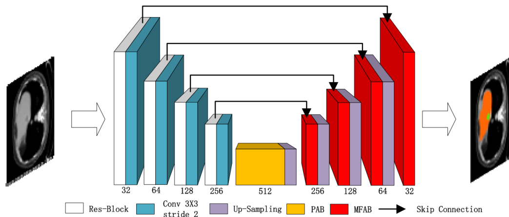
圖 4.2 MA-Net 架構(Fan et al., 2020)
