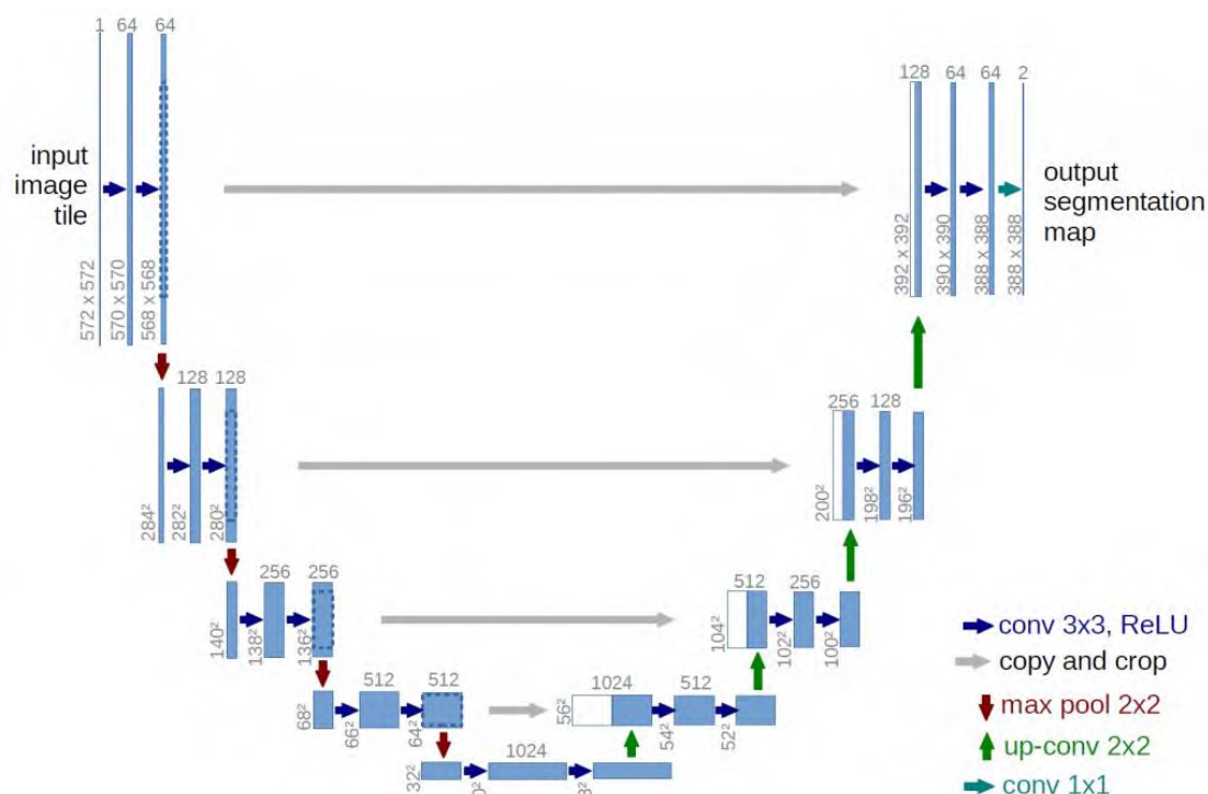
圖 4.1 Unet 架構
