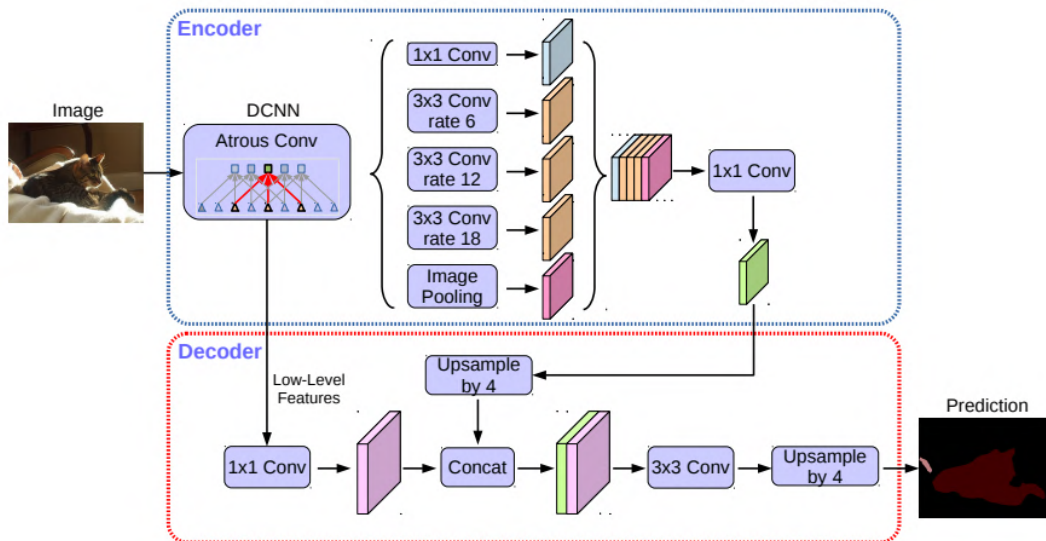
圖 4.4 DeepLabV3Plus 架構
