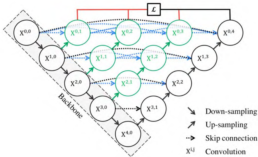
圖 4.3 U-Net++架構( Zhou et al.,2018)
